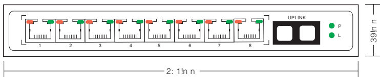
后面板视图
